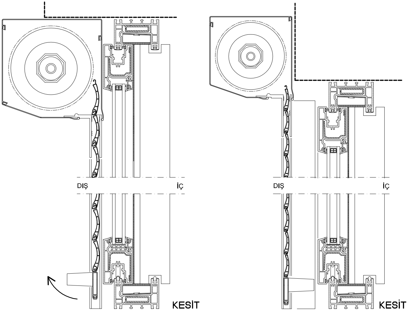
DOĞRAMAYA MONTAJ
